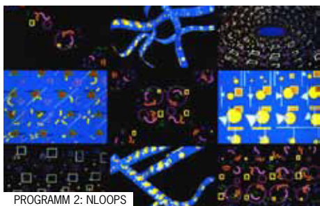
PROGRAMM 2: NLOOPS
